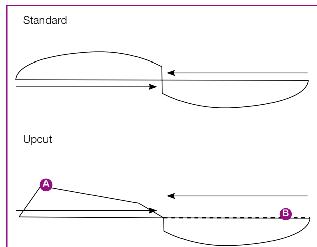
A Lame supérieure rasoir B Lame inférieure crantée
